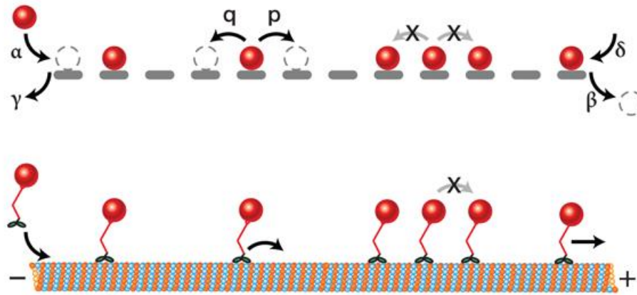
Open ASEP
